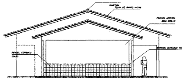
3 VISTA 3 ESCALA 1/50
