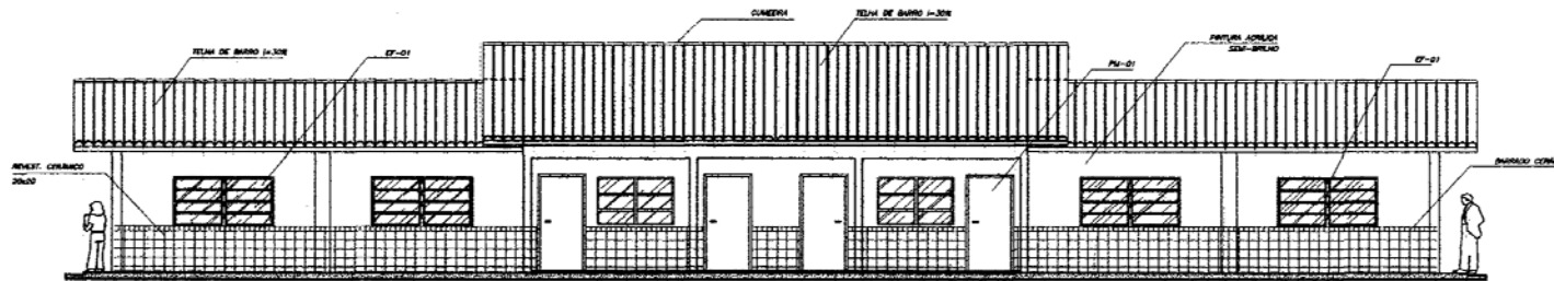
1 VISTA 1 ESCALA 1/50
