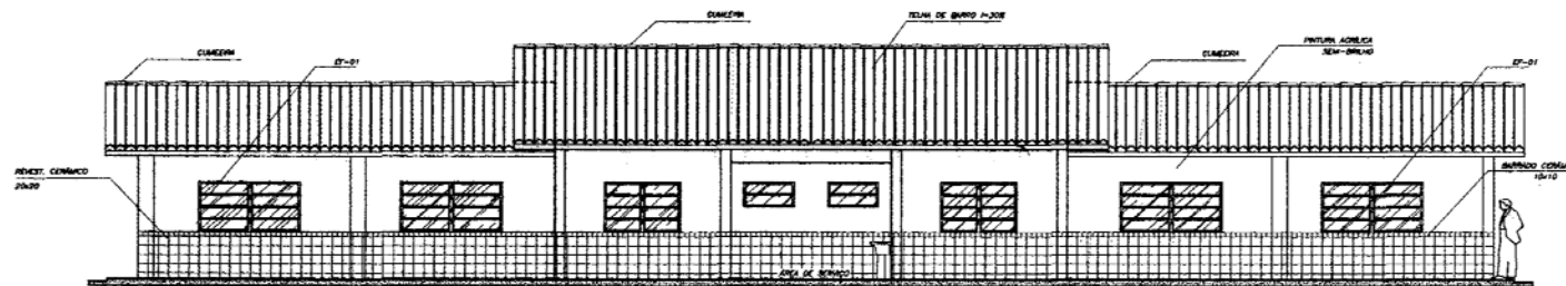
2 VISTA 2 ESCALA 1/50
