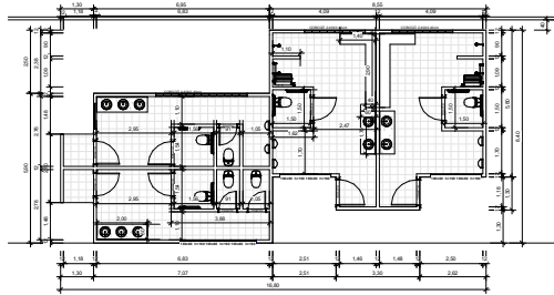
1 PLANTA BAIXA 1 : 100
