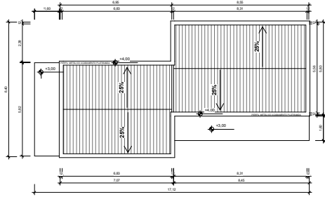
2 COBERTURA 1 : 100
