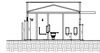
7 BB 1 : 75
